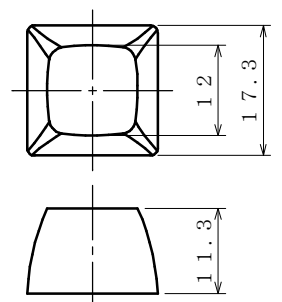
キートップ(QTT)寸法図
