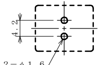
プリント基板穴加工図
