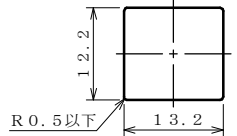
スイッチ取付穴加工図
